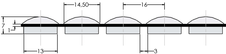
Perçin Birleştirmeli Alüminyum Palet - ALP3 (Bombeli)
