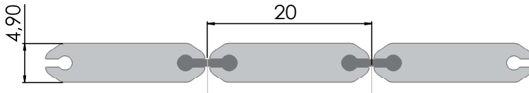
Kauçuk Fitilli Alüminyum Palet - ALP 2
