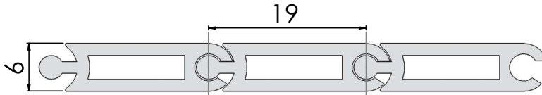
Geçmeli Alüminyum Palet - ALP1
